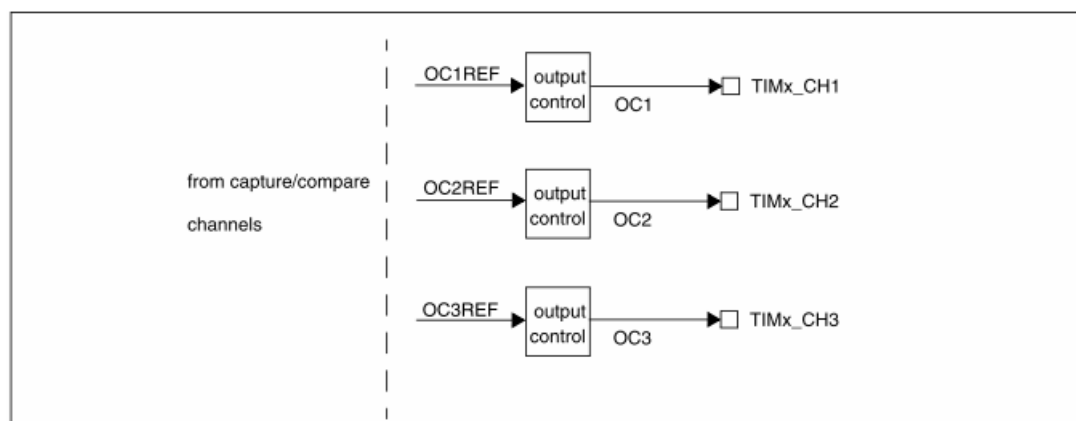
图84 输出部分框图
