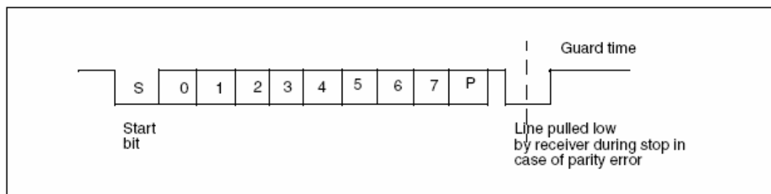
图112 ISO7816-3异步协议
